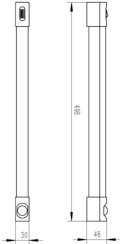
外形尺寸图纸
